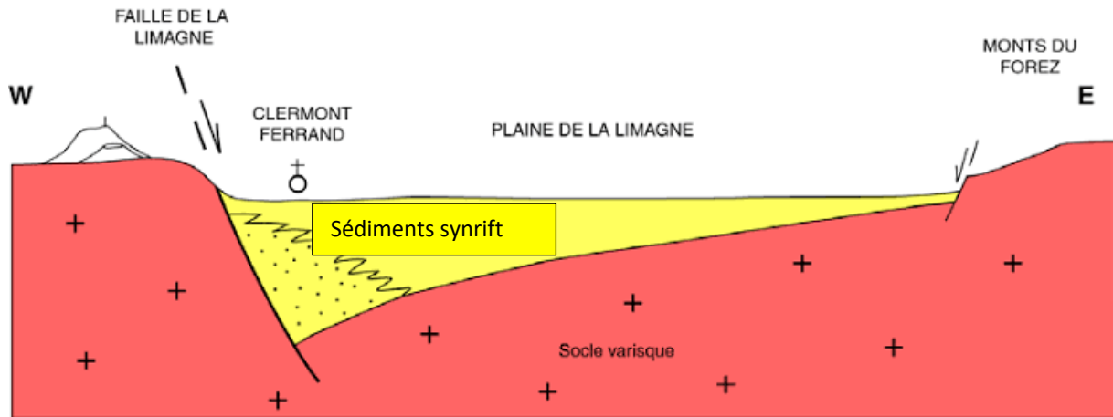
Disposition des sédiments synrift au niveau de la plaine de la Limagne
