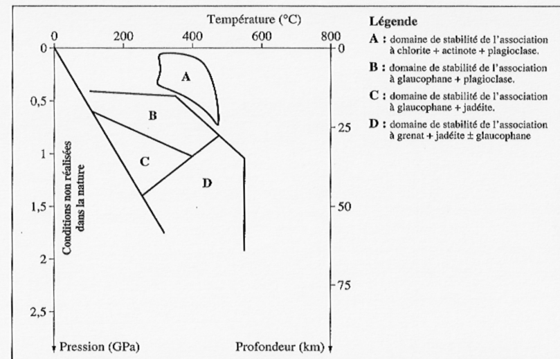
DOCUMENT 1 B. Diagramme pression-température représentant les domaines de stabilité des minéraux présents dans les roches métamorphiques.
